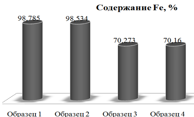
Рисунок – Содержание железа в исследуемых образцах деталей
