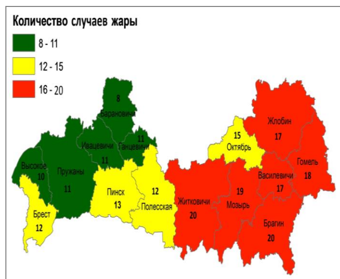
Рисунок 3 – Зонирование территории Белорусского Полесья по количеству случаев проявления сильной жары
