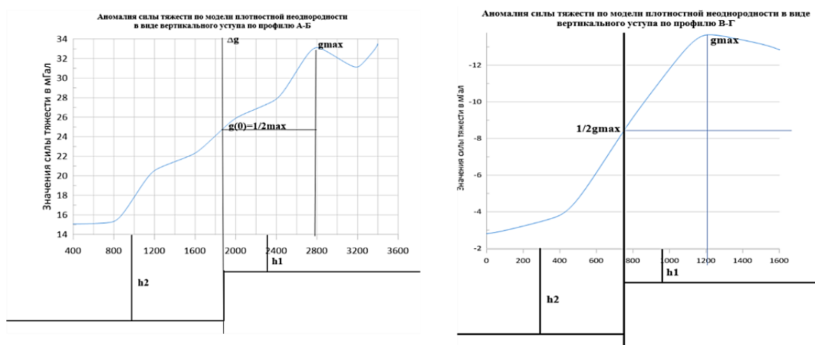
Рисунок 2 – Решение обратной задачи гравиразведки для вертикального уступа по профилям (составлено автором)
