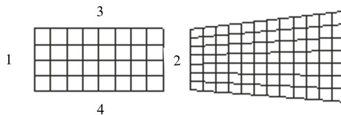
Рисунок 4 – Четырехугольники с разбивкой на элементы
