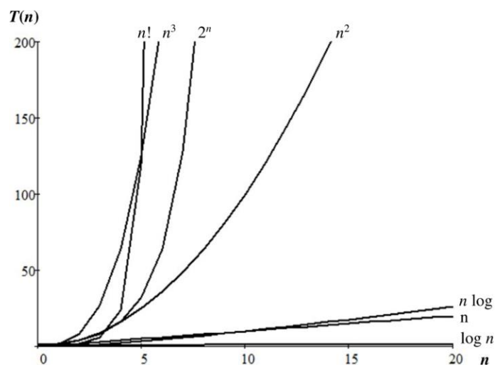
Рисунок – Сравнение эффективности алгоритмов различных классов
