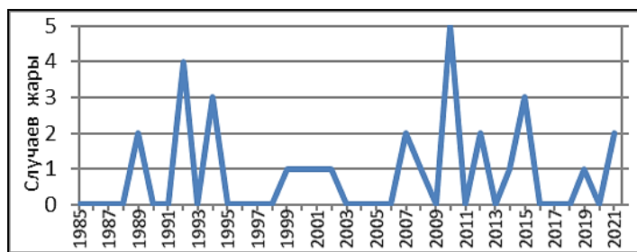
Рисунок 1а – Распределение количества случаев жары за 1985-2021 гг.
