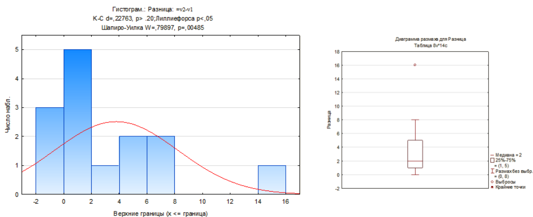
Рисунок 1 – Частотная и ящечная гистограмма нормальности распределения данных
